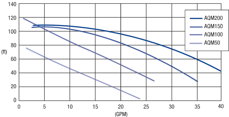
Curva de operación de la bomba
